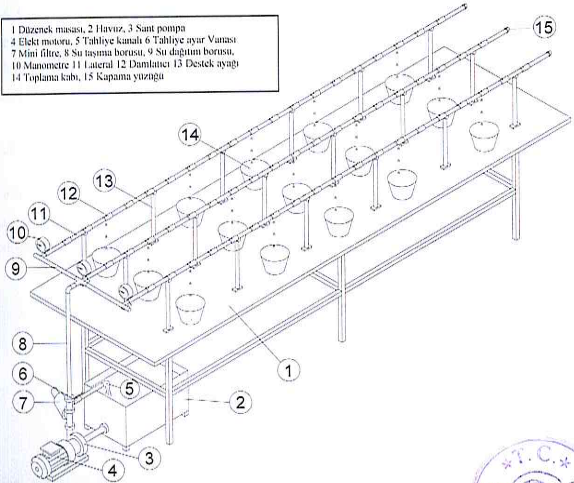
Şekil 2. Ölçümlerde kullanılan deney düzeneği
