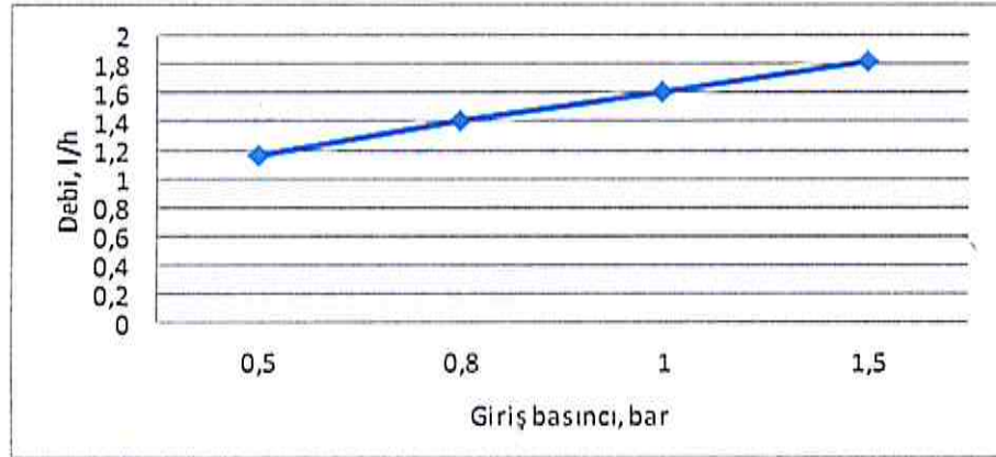
Şekil 3. Ardent Marka, 22 mm 1,6 l/h debili 30 cm damlatıcı aralıklı damla sulama borusuna ait giriş basıncı, debi değişimi
